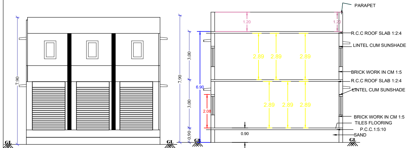
ELEVATION
