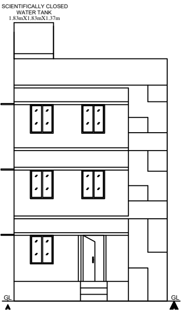
ELEVATION
