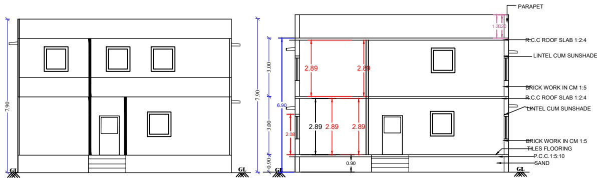
ELEVATION
