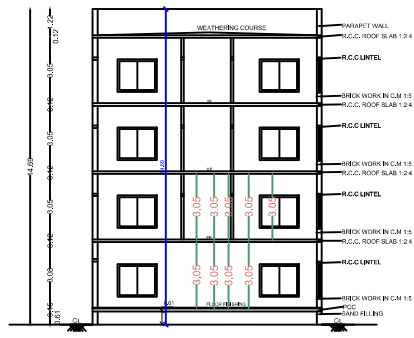
SECTION A-A1
