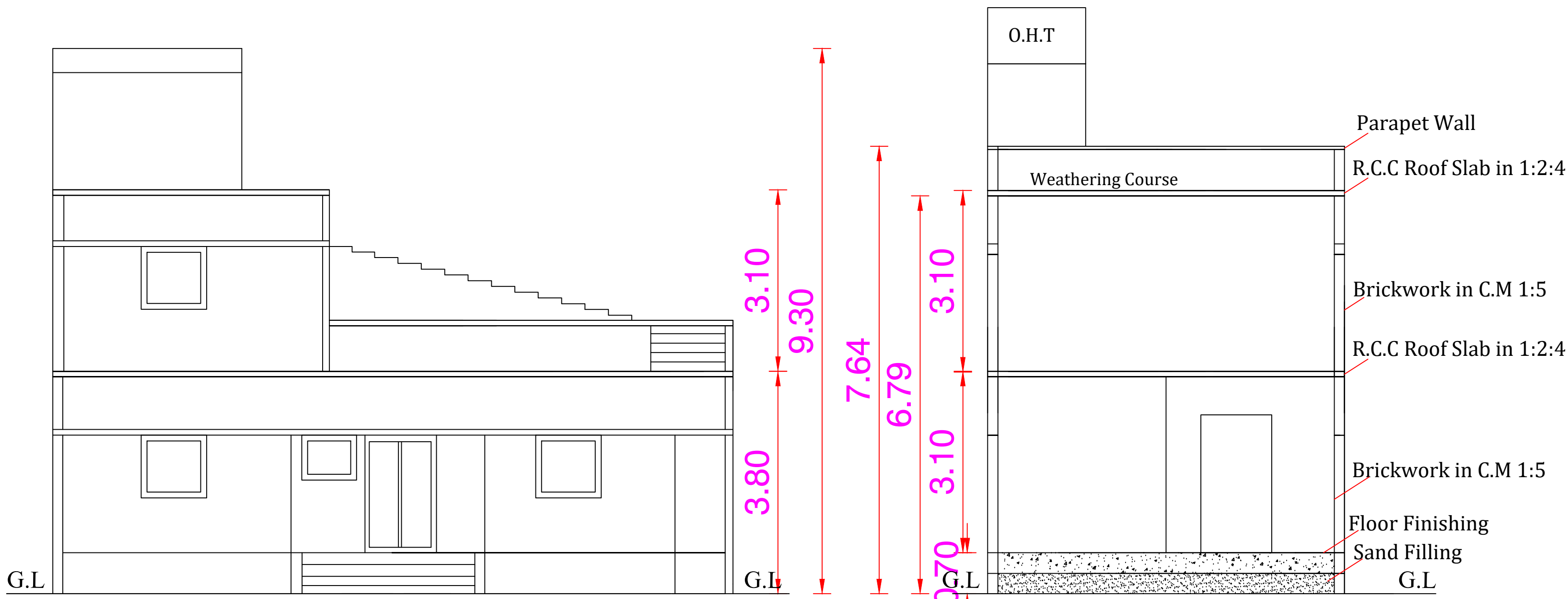
ELEVATION
