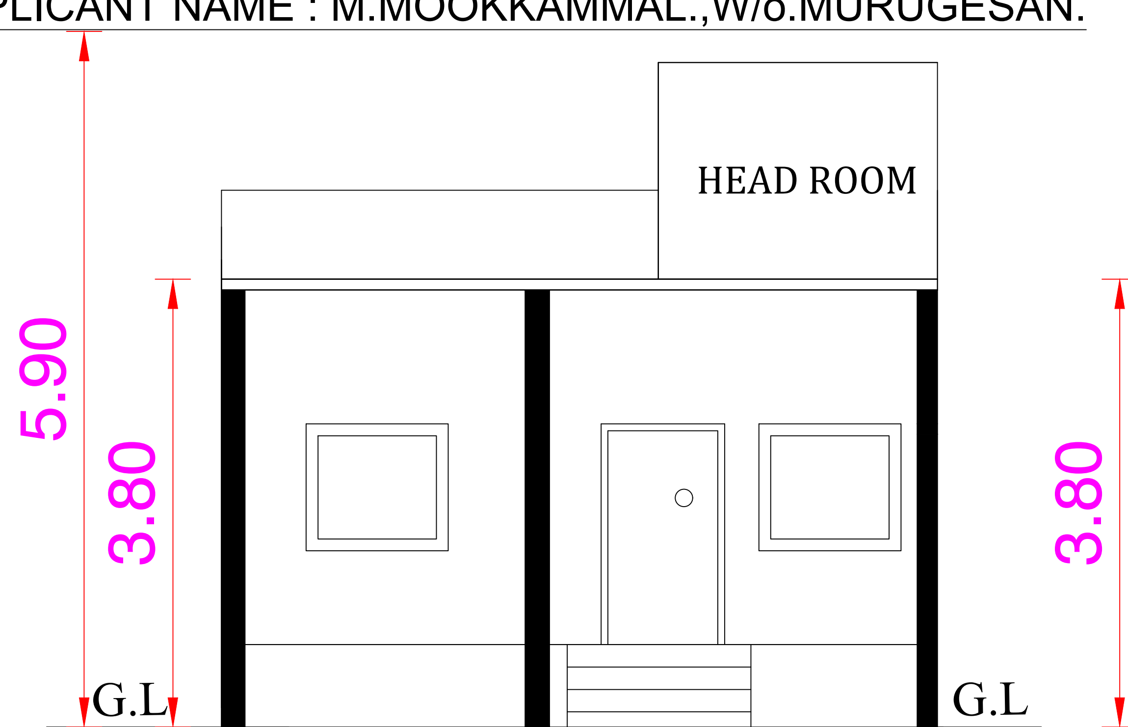
ELEVATION
