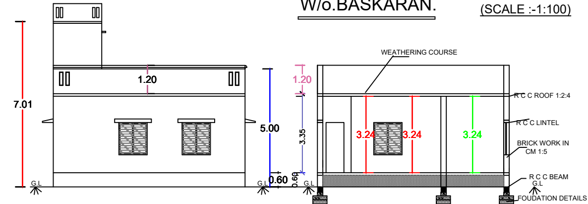
ELEVATION
