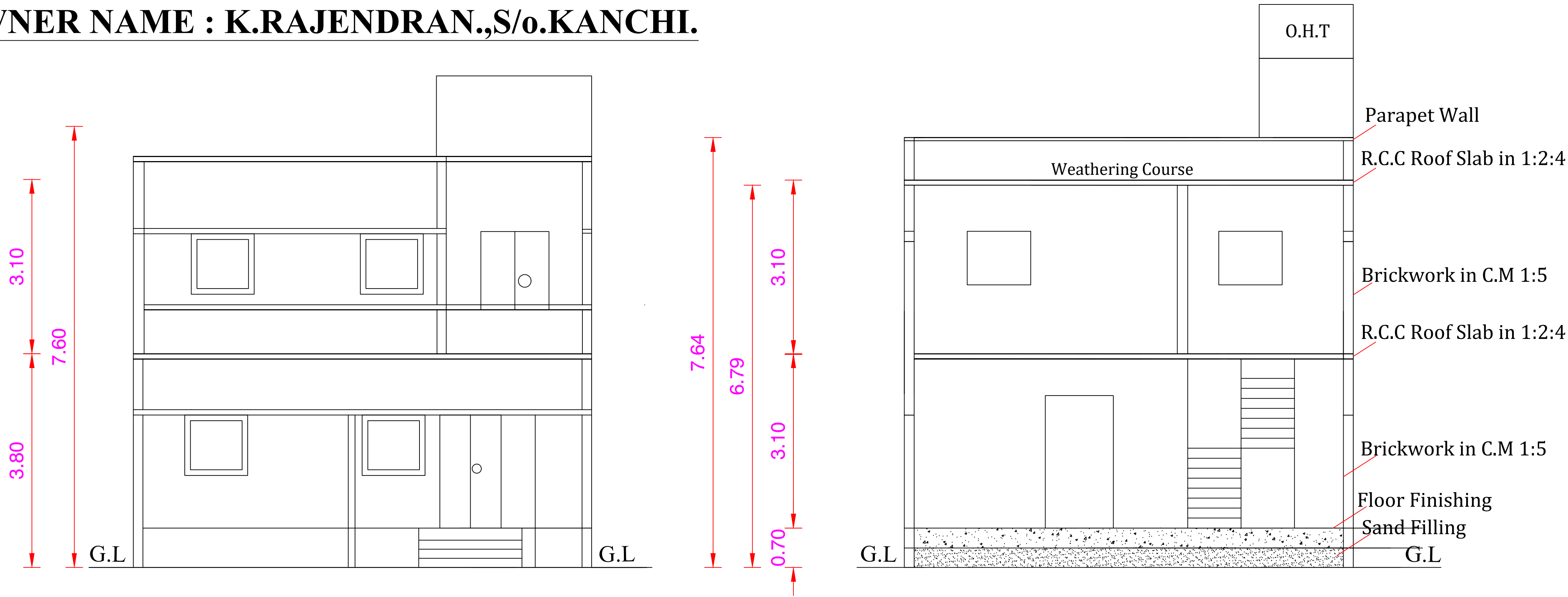
ELEVATION
