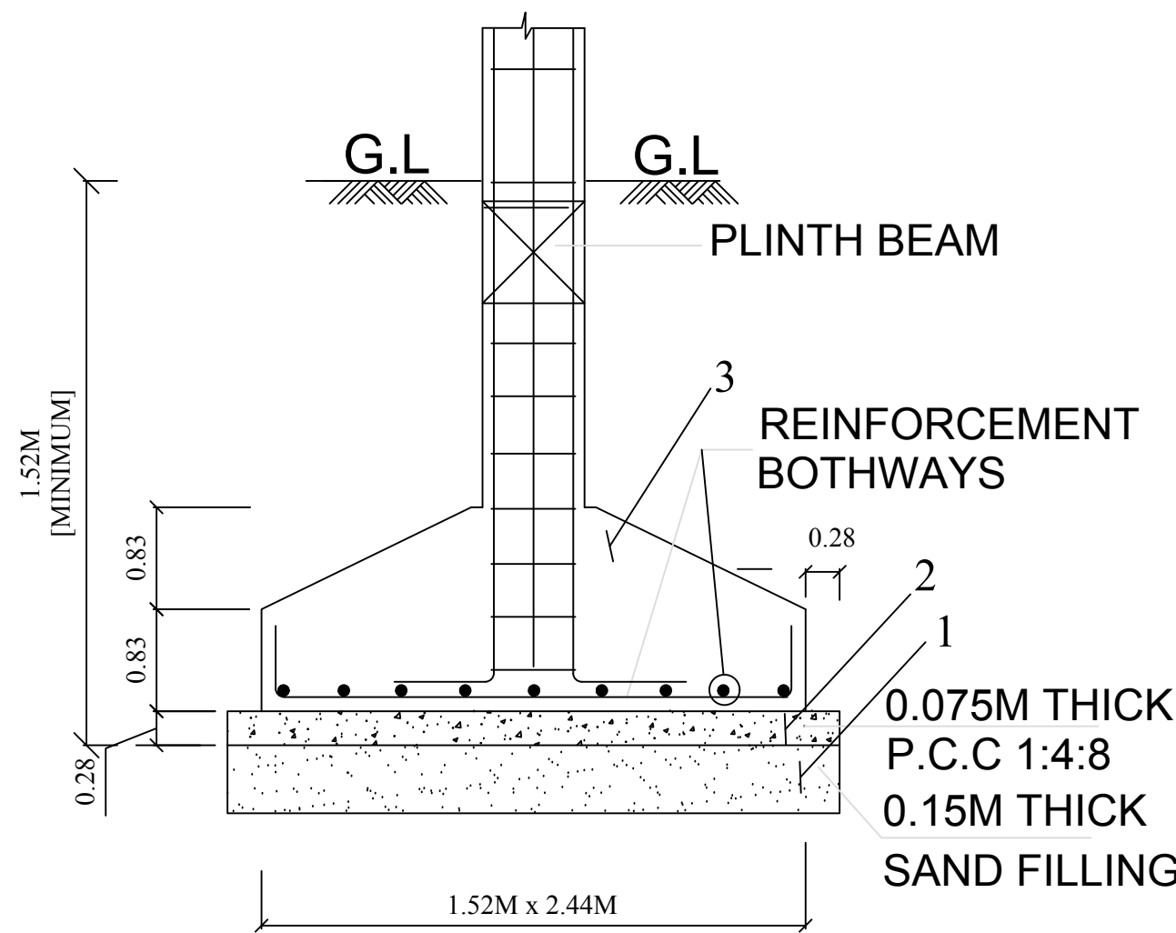
TYP. DET. COLUMN FOOTING
