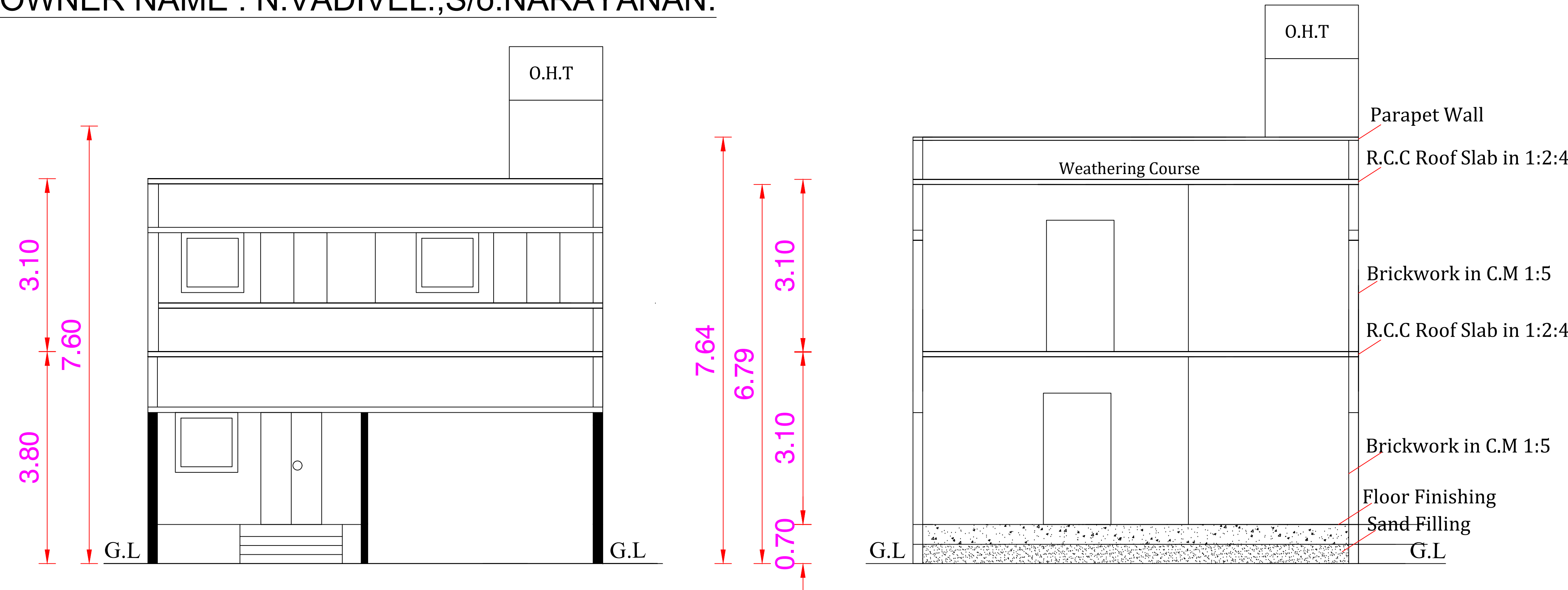
ELEVATION
