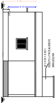
ELEVATION
