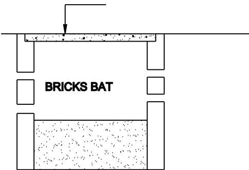
SOAK PIT
