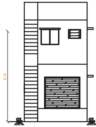
ELEVATION
