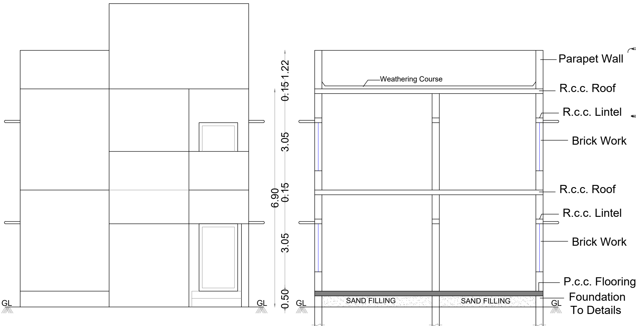
ELEVATION
