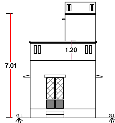
ELEVATION
