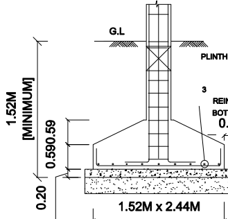
TYP. DET. COLUMN FOOTING
