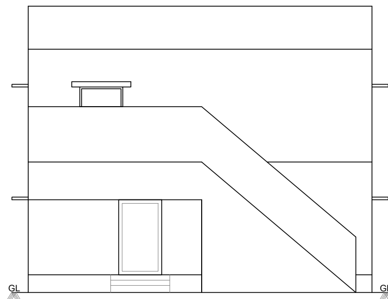
ELEVATION
