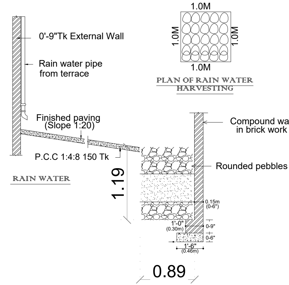
ELEVATION
