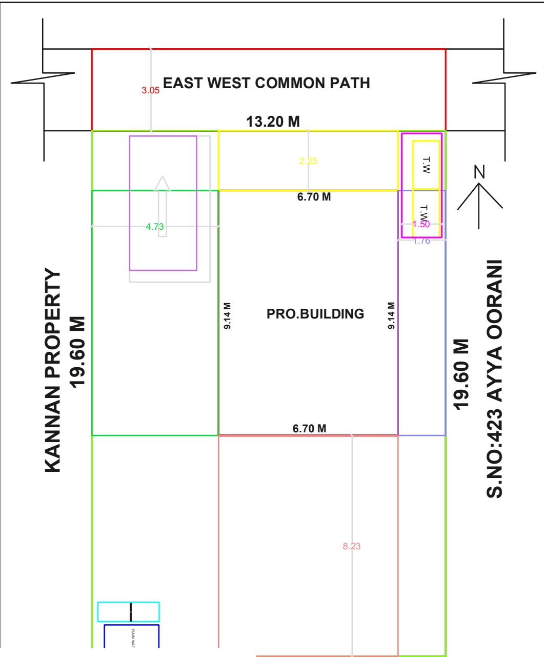
20 M ER PROPERTY SITE PLAN
