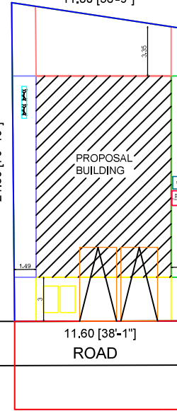
SITE PLAN Scale 1:100
