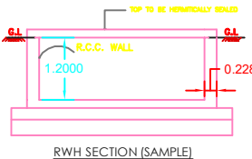
RWK_CAPACITY_L=2000LTRS
