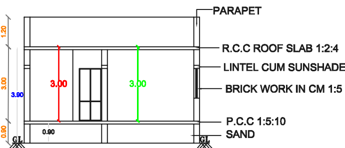
ELEVATION
