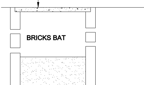
SOAK PIT
