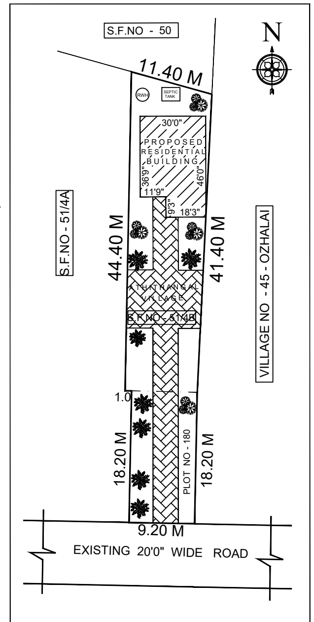
SITE PLAN SCALE 1:400
