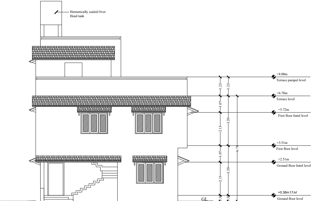
ELEVATION - A
