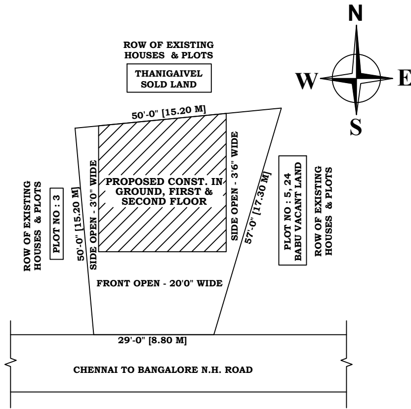
SITE PLAN:
