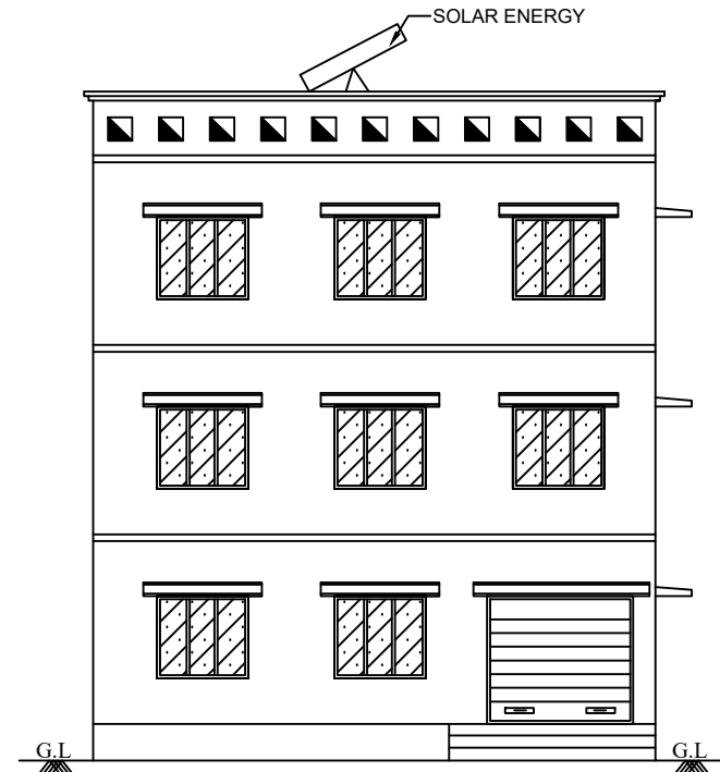
ELEVATION
