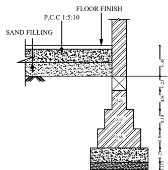
FOUNDATION DETAIL N.T.S
