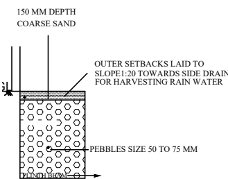
FOUNDATION DETAIL N.T.S
