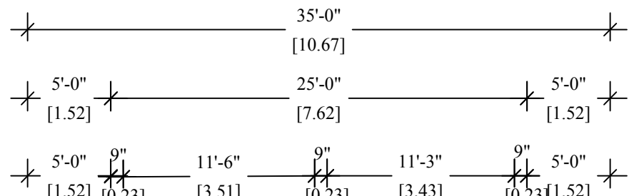
ELEVATION
