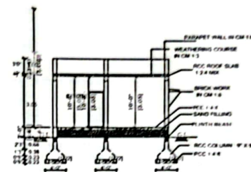
SECTION - AB
