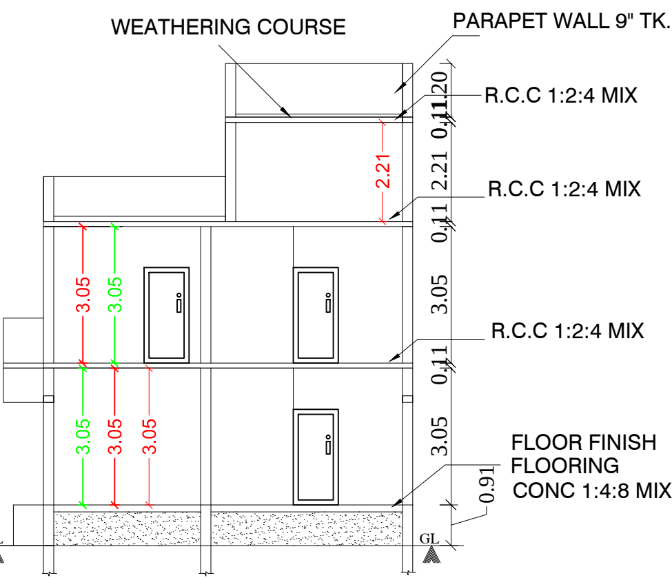
SECTION : "A-A" (SCALE: 1CM : 1M)
