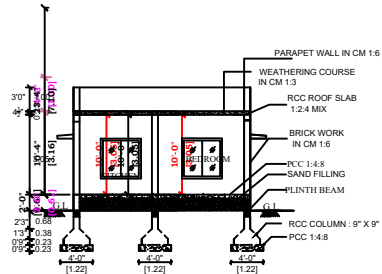
SECTION - AB
