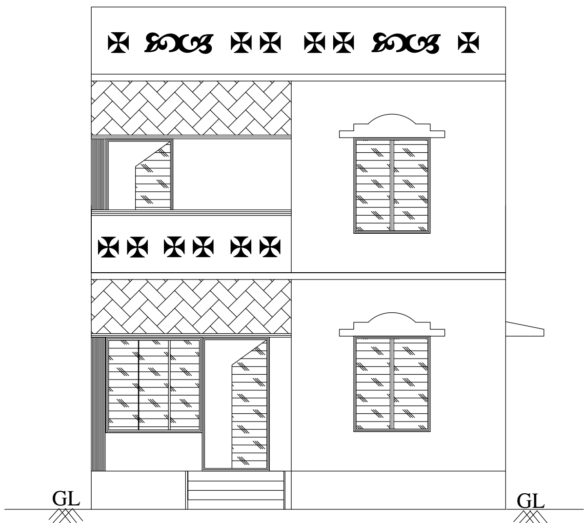
ELEVATION
