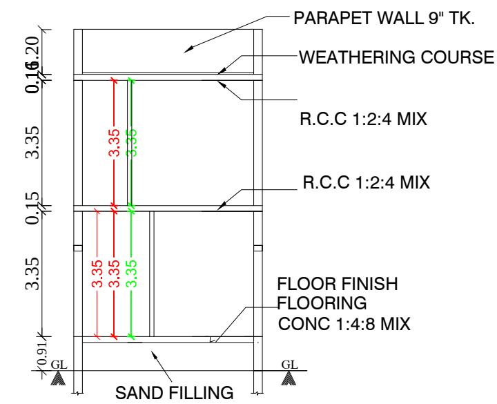
SECTION : "A-A" (SCALE: 1CM : 1M)
