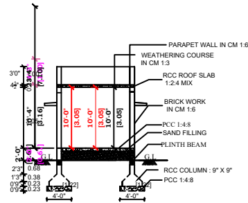
SECTION - AB
