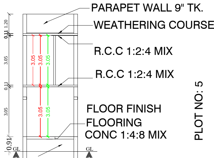
SECTION : "A-A" (SCALE: 1 CM : 1 M)
