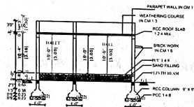
SECTION - AB
