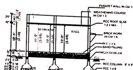
SECTION - AB
