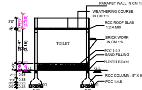
SECTION - AB
