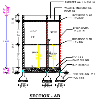
SECTION - AB
