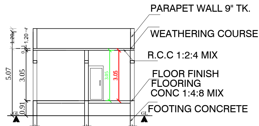
SECTION : "A-A" (SCALE: 1CM : 1M)
