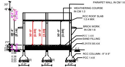
SECTION - AB
