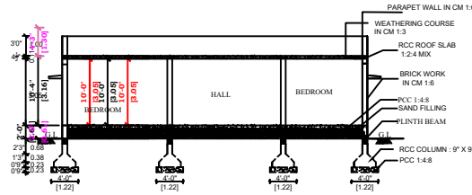
SECTION - AB
