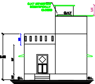
ELEVATION
