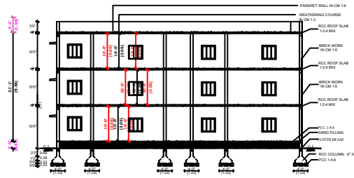
SECTION - AB
