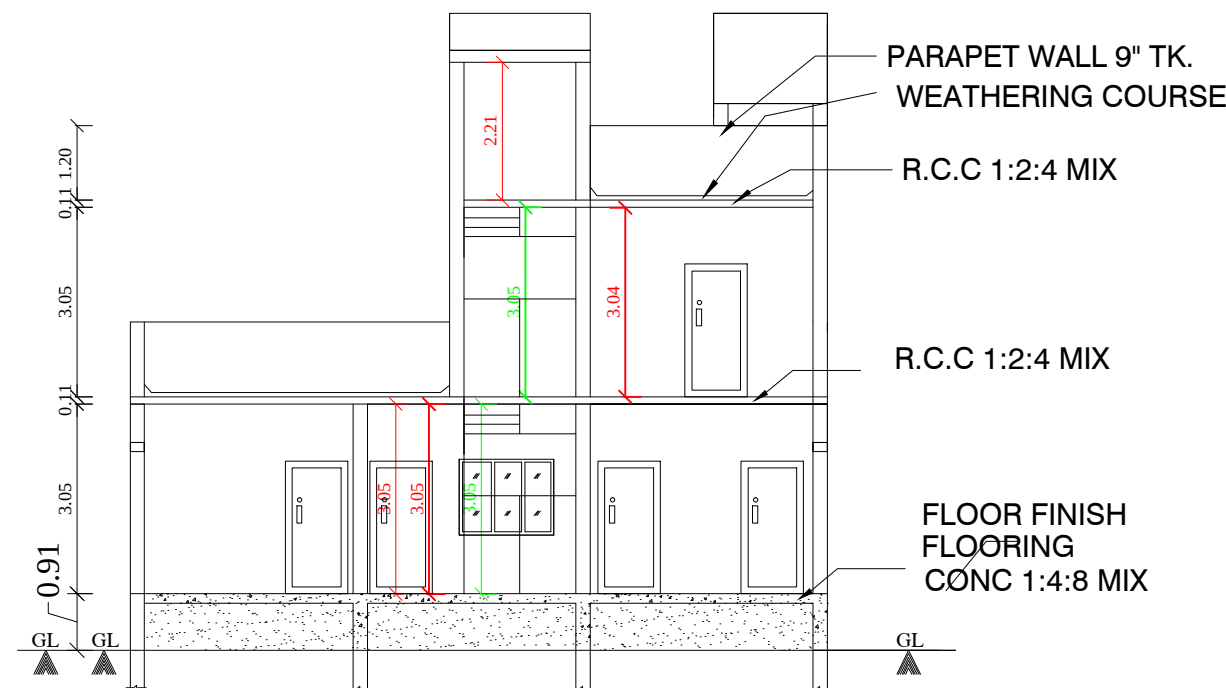
SECTION : "A-A" (SCALE: 1CM : 1M)
