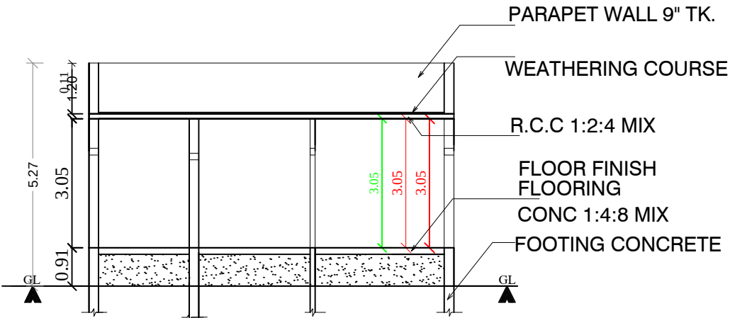
SECTION : "A-A" (SCALE: 1CM : 1M)
