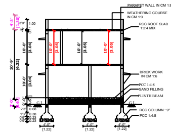
SECTION - AB
