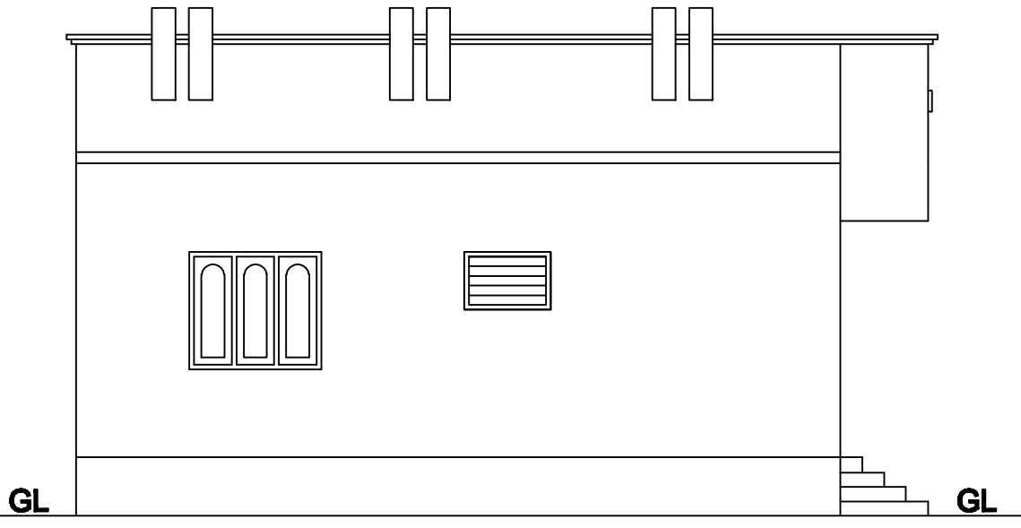
ELEVATION
