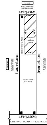
SITE PLAN: SCALE: 1:200
