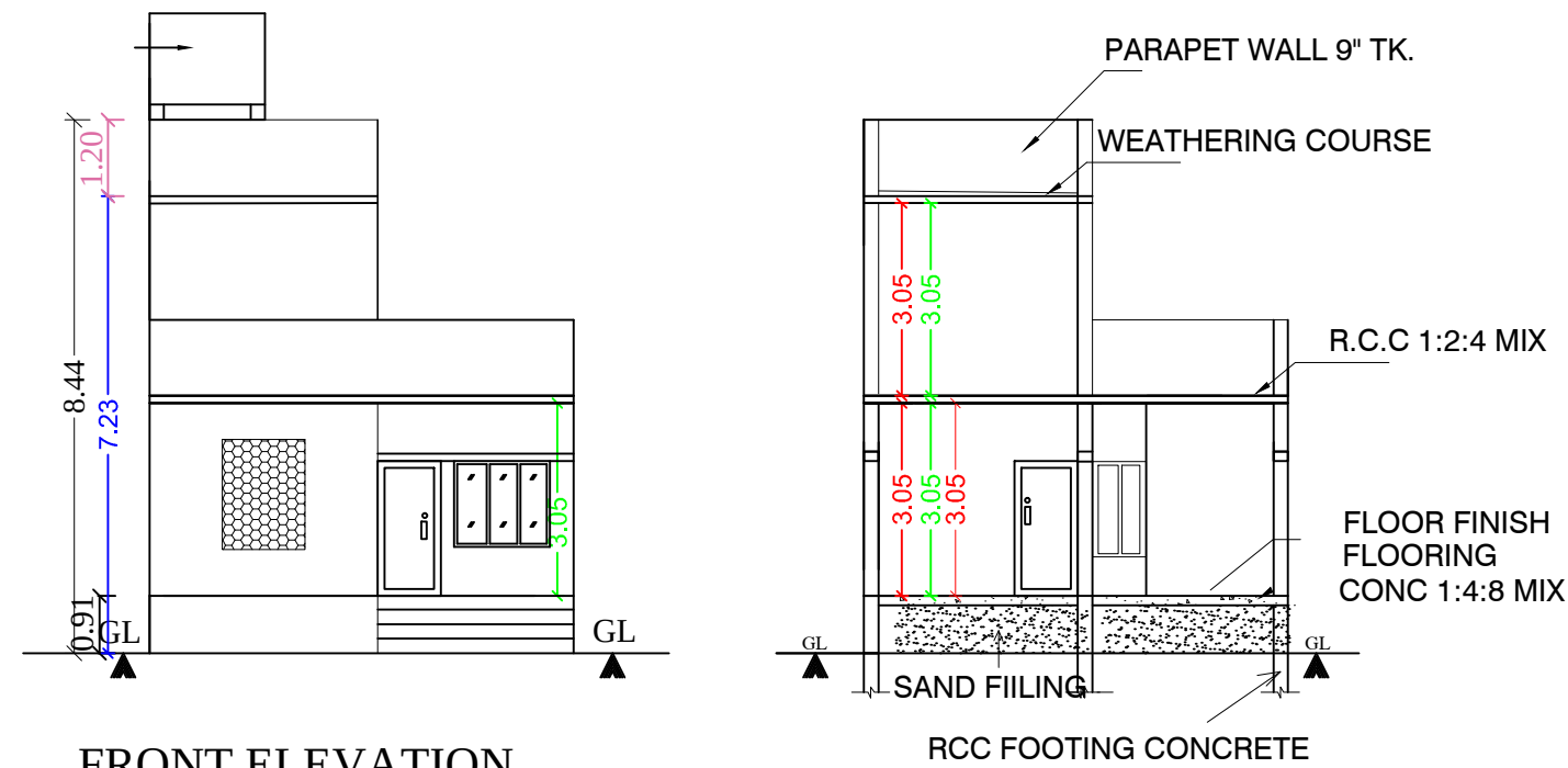
SECTION : "A-A" (SCALE: 1CM : 1M)
